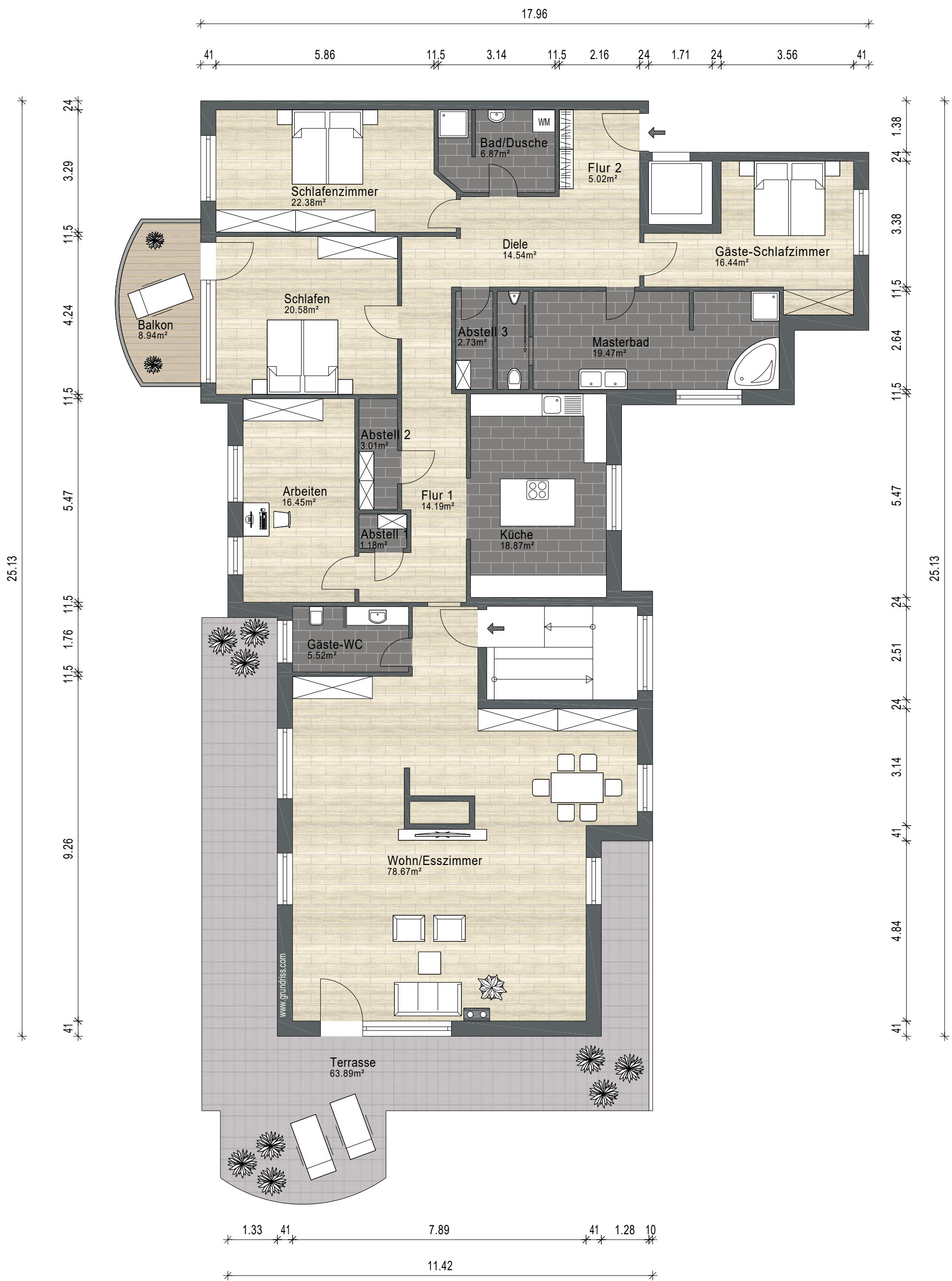
1.Obergeschoss
